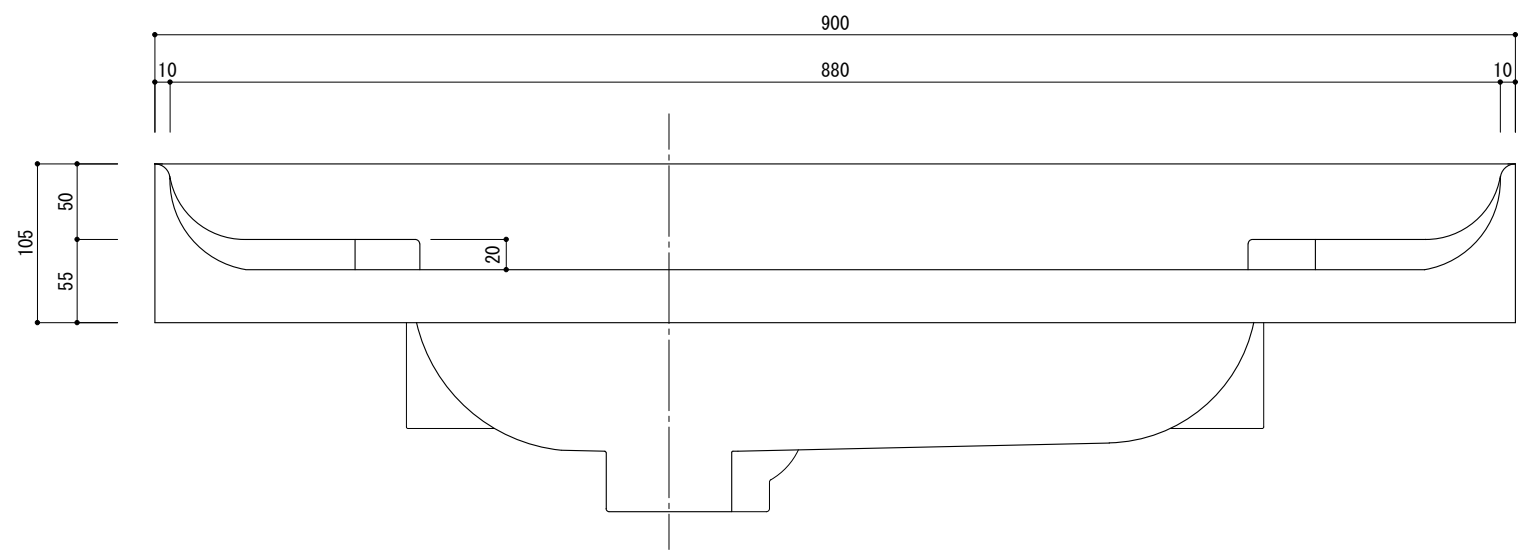
正面図 (S=1/5)
