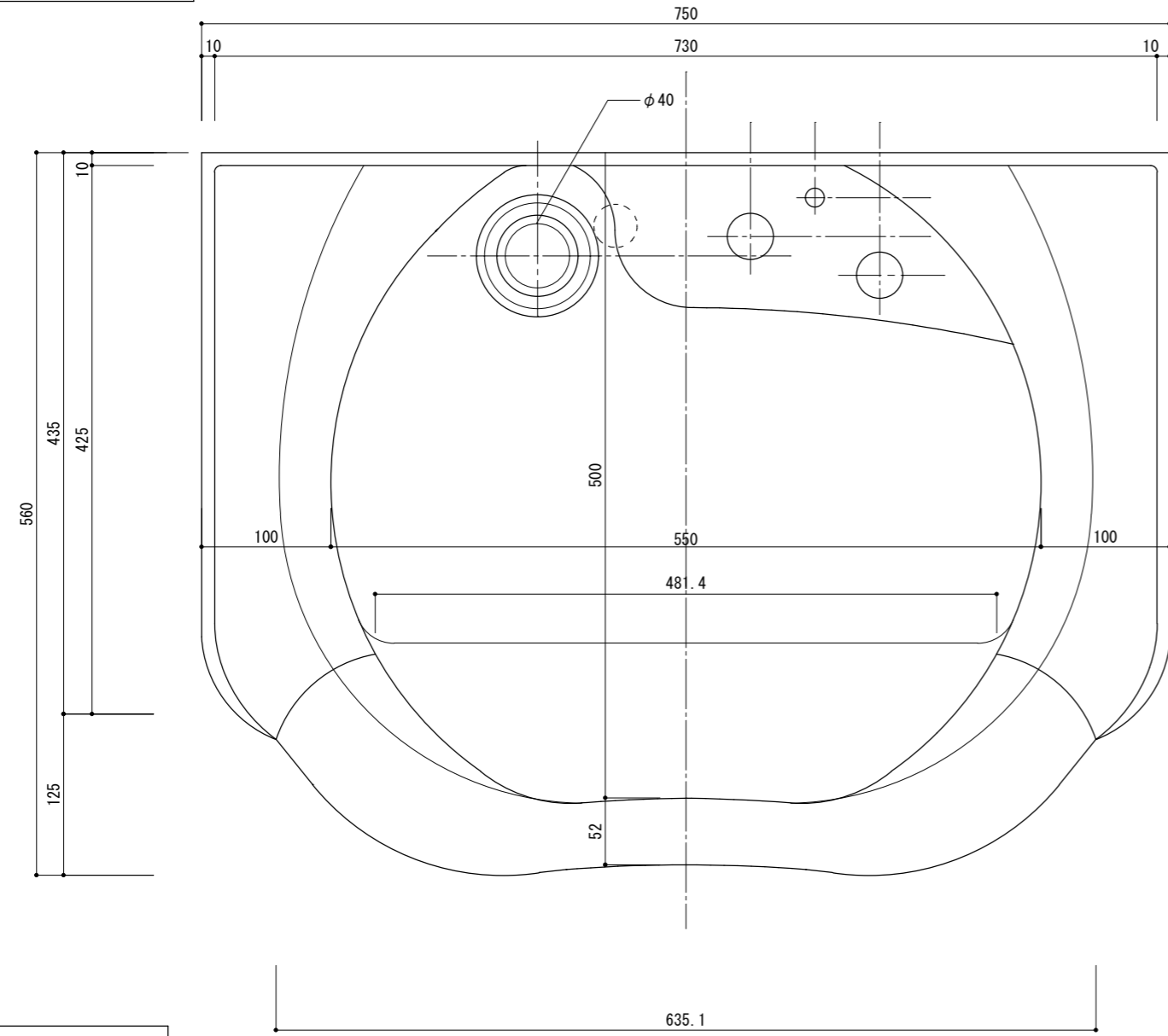
正面図 (S=1/5)
