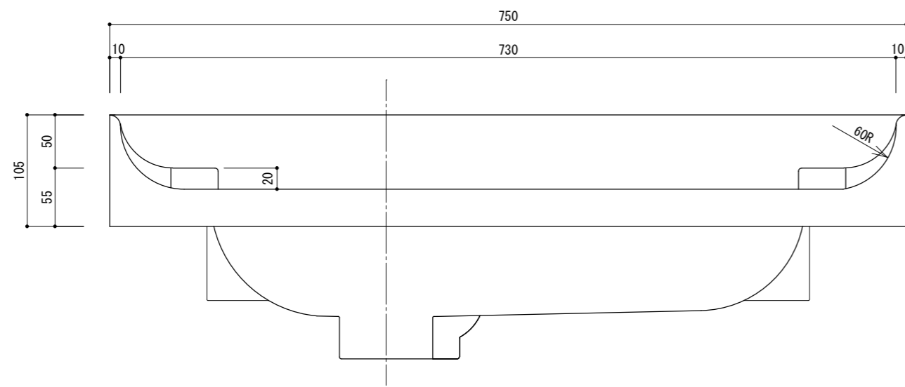
正面図 (S=1/5)
