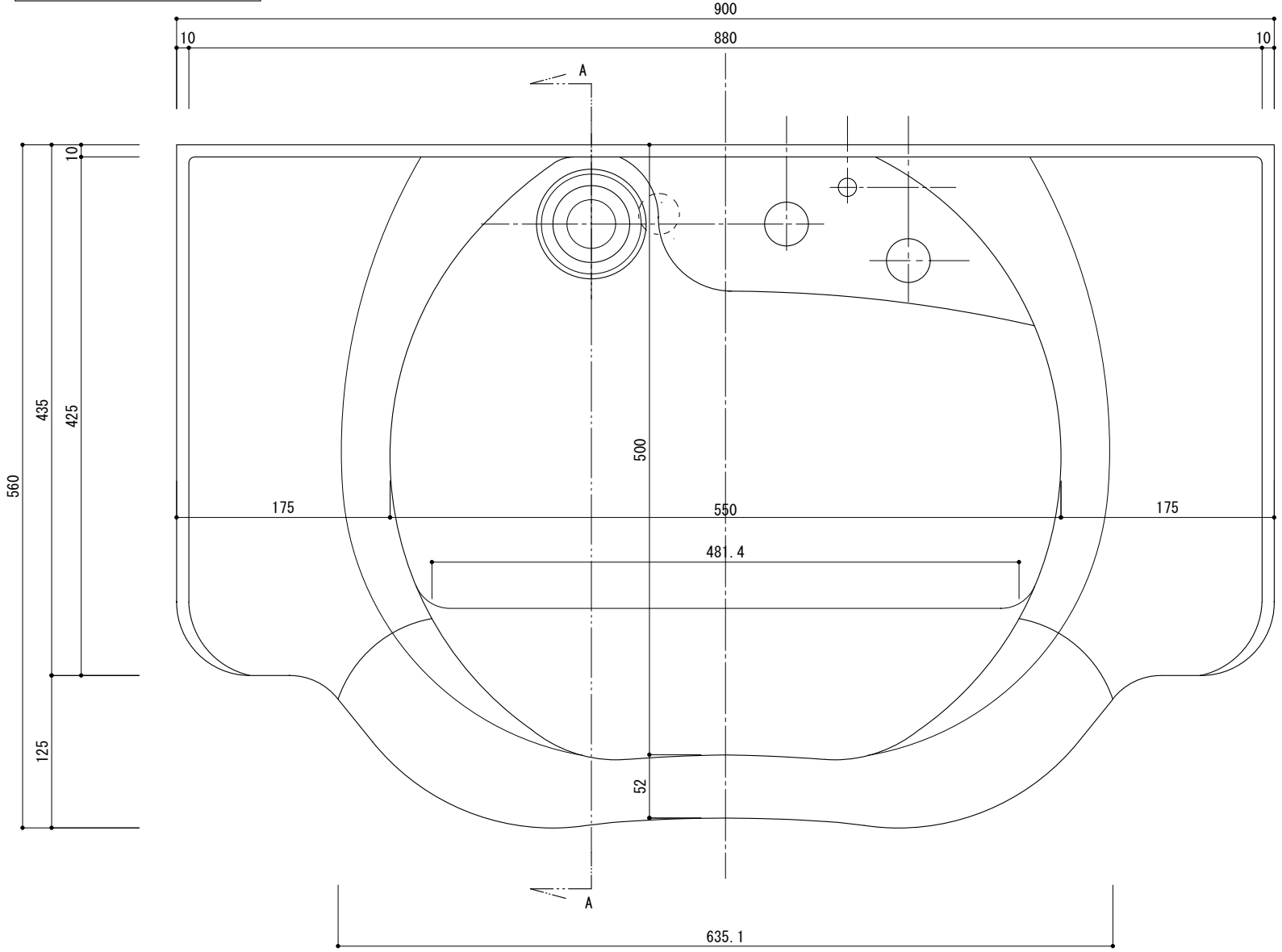
正面図 (S=1/5)
